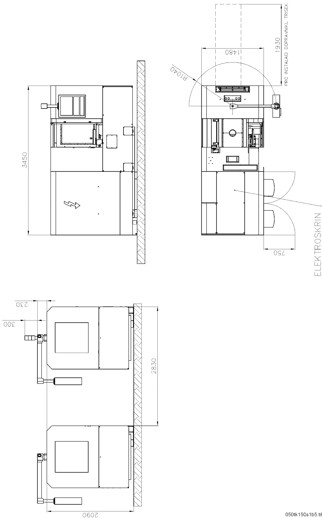
Obr. 1.4-5: Hlavní rozměry stroje s dopravníkem třísek se skrytou výspnou částí
