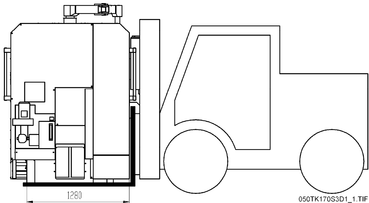
Obr. 3.2.2-1: Zvedání stroje vysokozdvižným vozíkem - pohled boční
