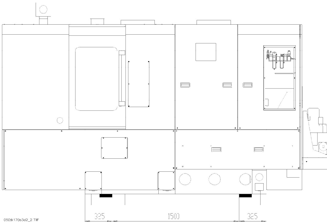
Obr. 3.2.2-2: Zvedání stroje vysokozdvižným vozíkem - pohled čelní
