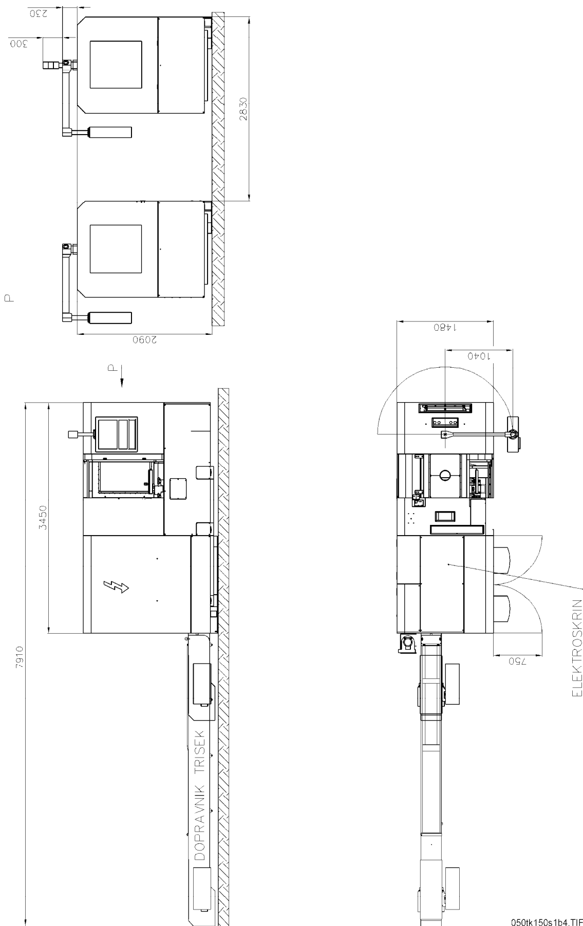
Obr. 1.4-3: Hlavní rozměry stroje s dopravníkem třísek bez zvýšené výsypné části – varianta 1
