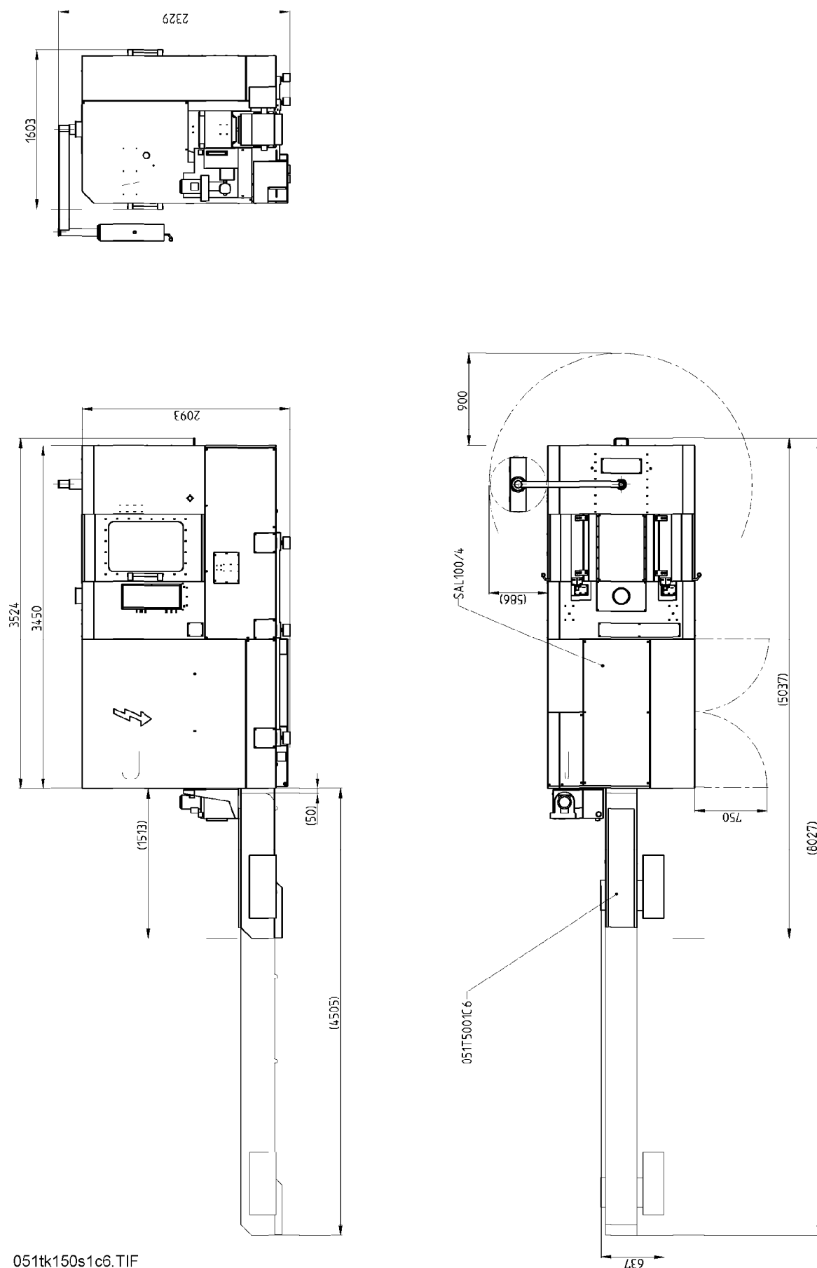
Obr. 1.4-4: Hlavní rozměry stroje s dopravníkem třísek bez zvýšené výsypné části – varianta 2
