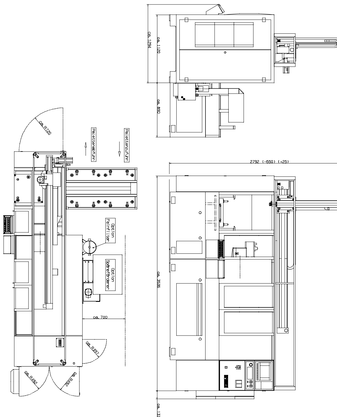
Abbildung 5-2: Aufstellplan PD mit Portallader
