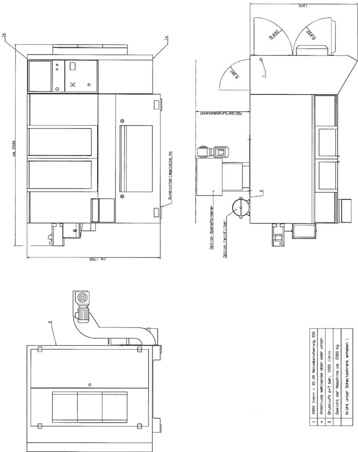
Abbildung 5-1: Aufstellplan
