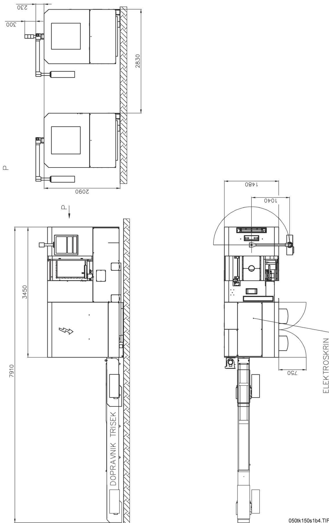
Obr. 1.4-2: Hlavní rozměry stroje s dopravníkem třísek bez zvýšené výsypné části
