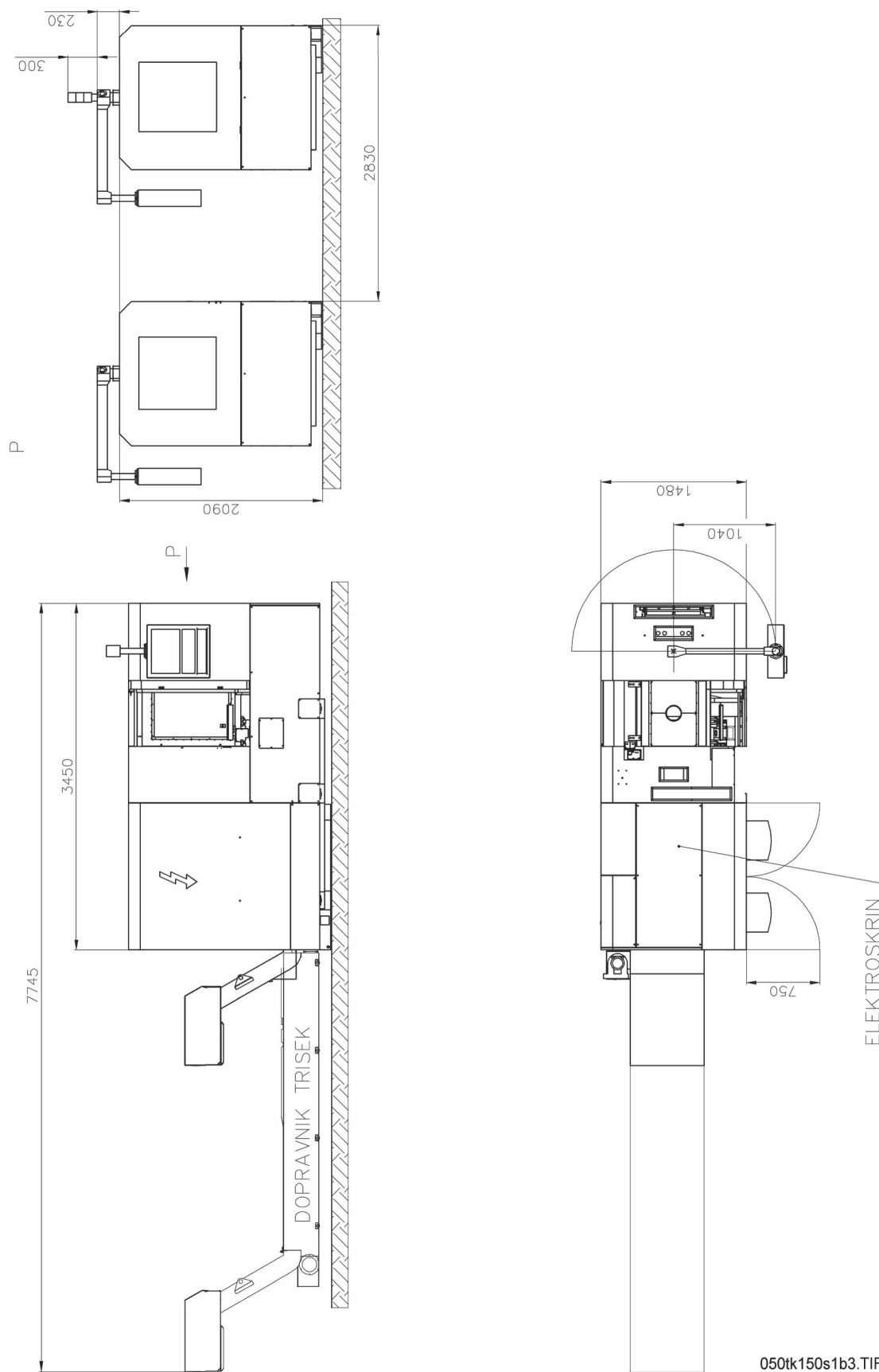
Obr. 1.4-1: Hlavní rozměry stroje s dopravníkem třísek se zvýšenou výsypnou částí
