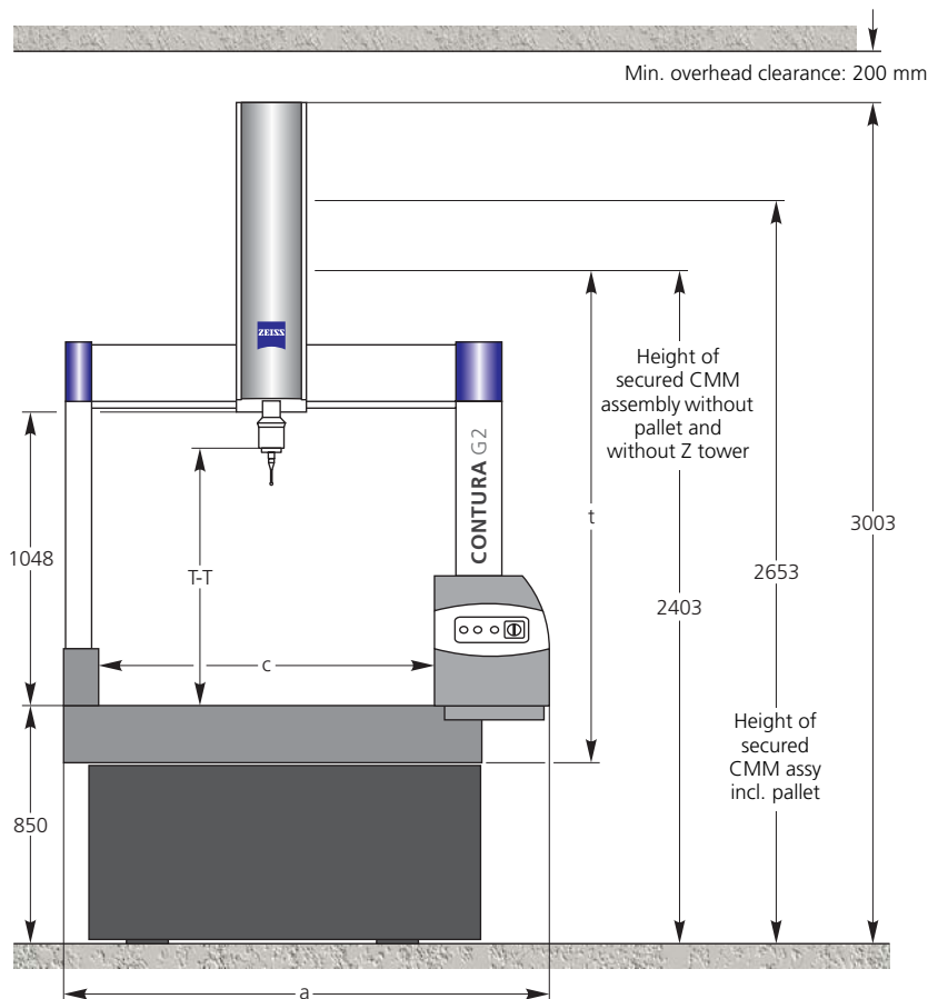
CONTURA G2 with optional U-profile
